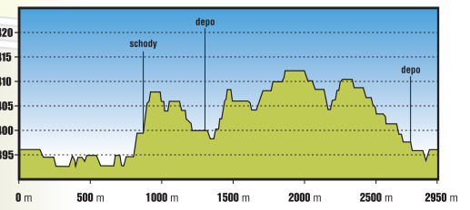
VÝŠKOVÝ PROFIL TRATĚ
